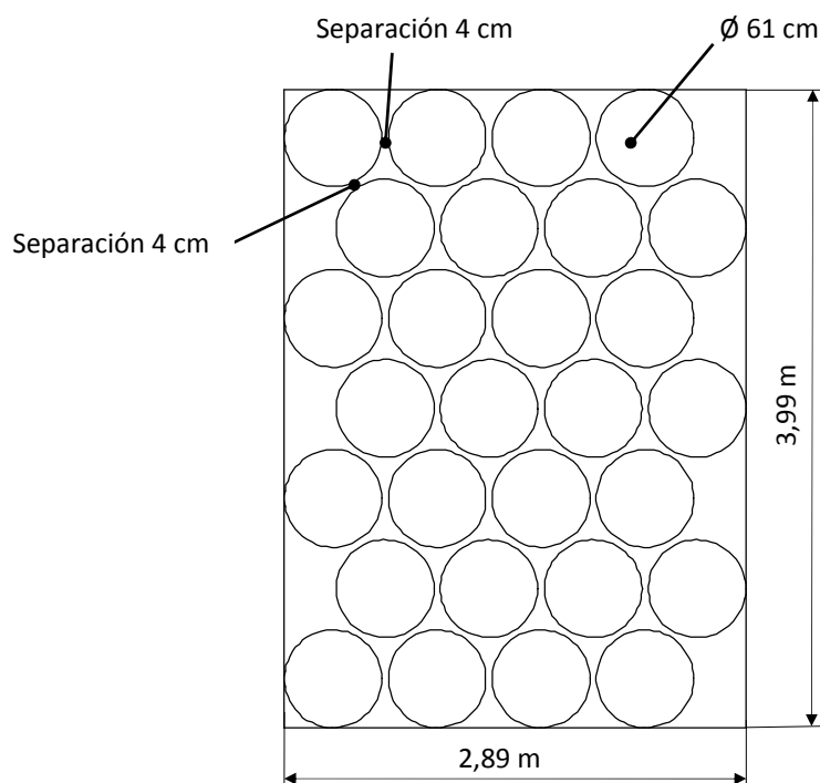
Figura 1: Disposición de muestra ensayada (B2017-30-M451)
