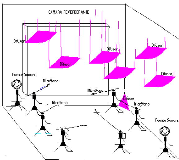
Figura 2: Esquema de la cámara reverberante
